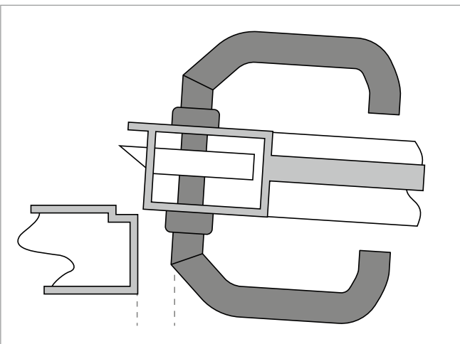
Abb. 23 gekrümmter Türgriff
