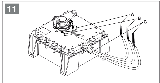
Anschluss MOTOR 1 (im Beispiel Rechts) an der Motorsteuerung MS1000
