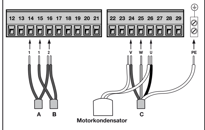
Anschluss MOTOR 2 (im Beispiel Links) an der Motorsteuerung MS1000
